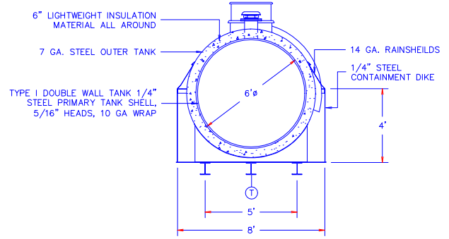
TANK SECTION A-A SCALE: 1"=5'
