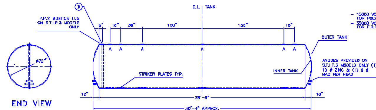
ELEVATION
